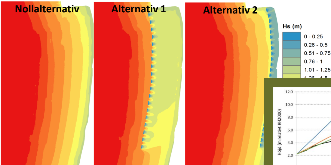
Signifikant våghöjd (Hs) för de tre simulerade alternativen.
